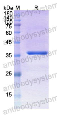
SDS-PAGE
