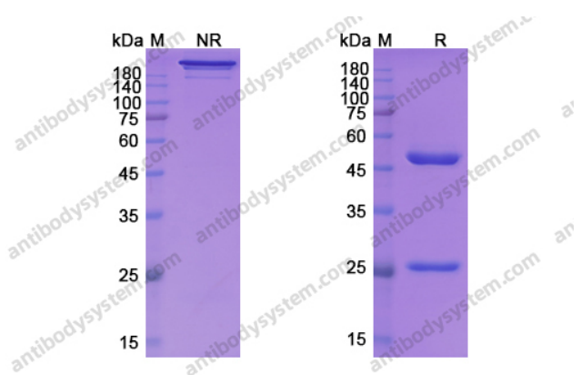
SDS-PAGE
